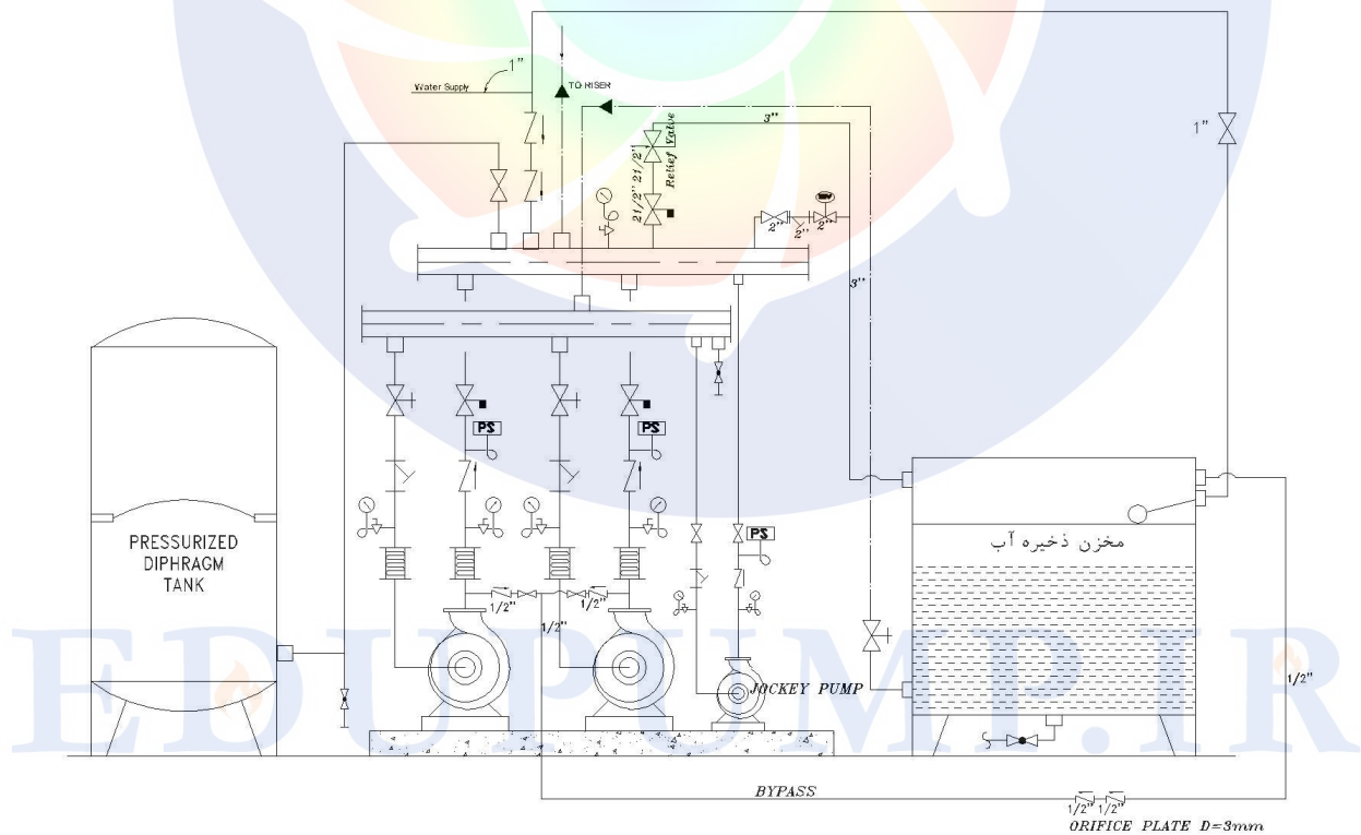
شکل ۱ (ب): نمای شماتیک مجموعه پمپ نمونه به همراه متعلقات (مخزن مشترک)
